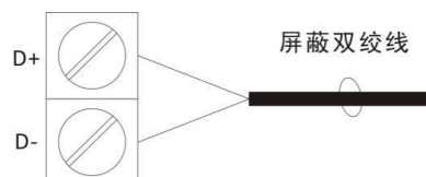
图 3-8 通信接线
