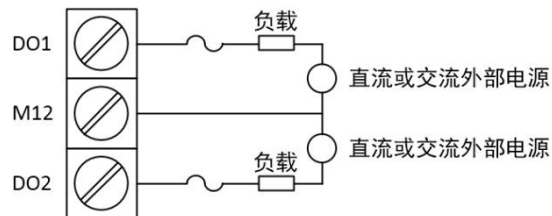
图 3-10 DO 接线示意图
