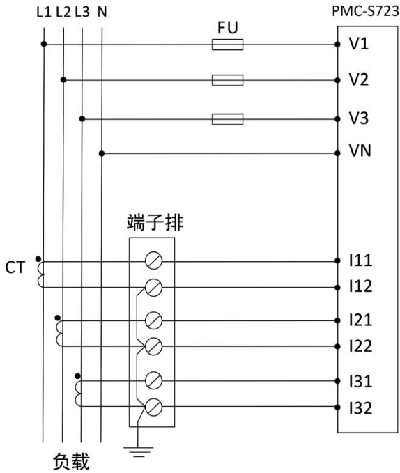
图 3-4 WYE, 无 PT, 3CT
