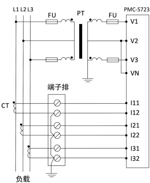
图 3-6 DELTA, 3CT
