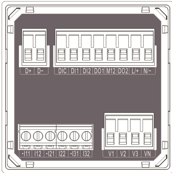
图 3-2 端子图 (2DI+2DO)
