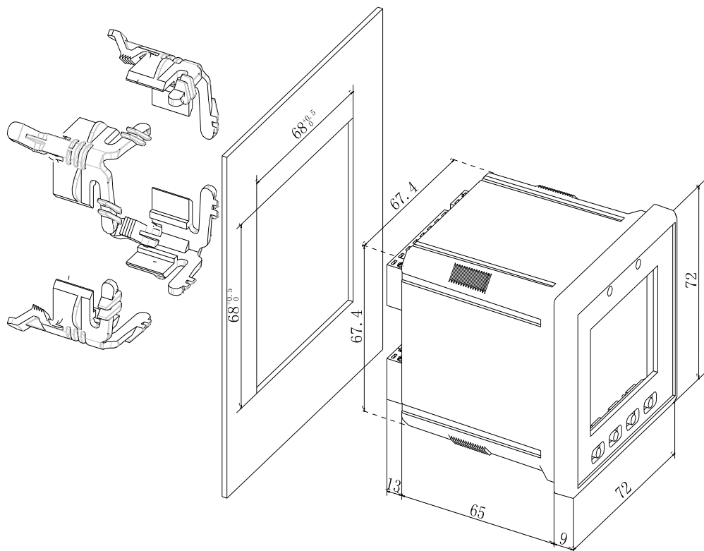
图 3-1 安装尺寸图
