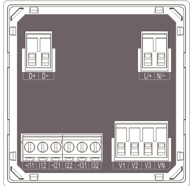
图 3-3 端子图 (无 I/O)
